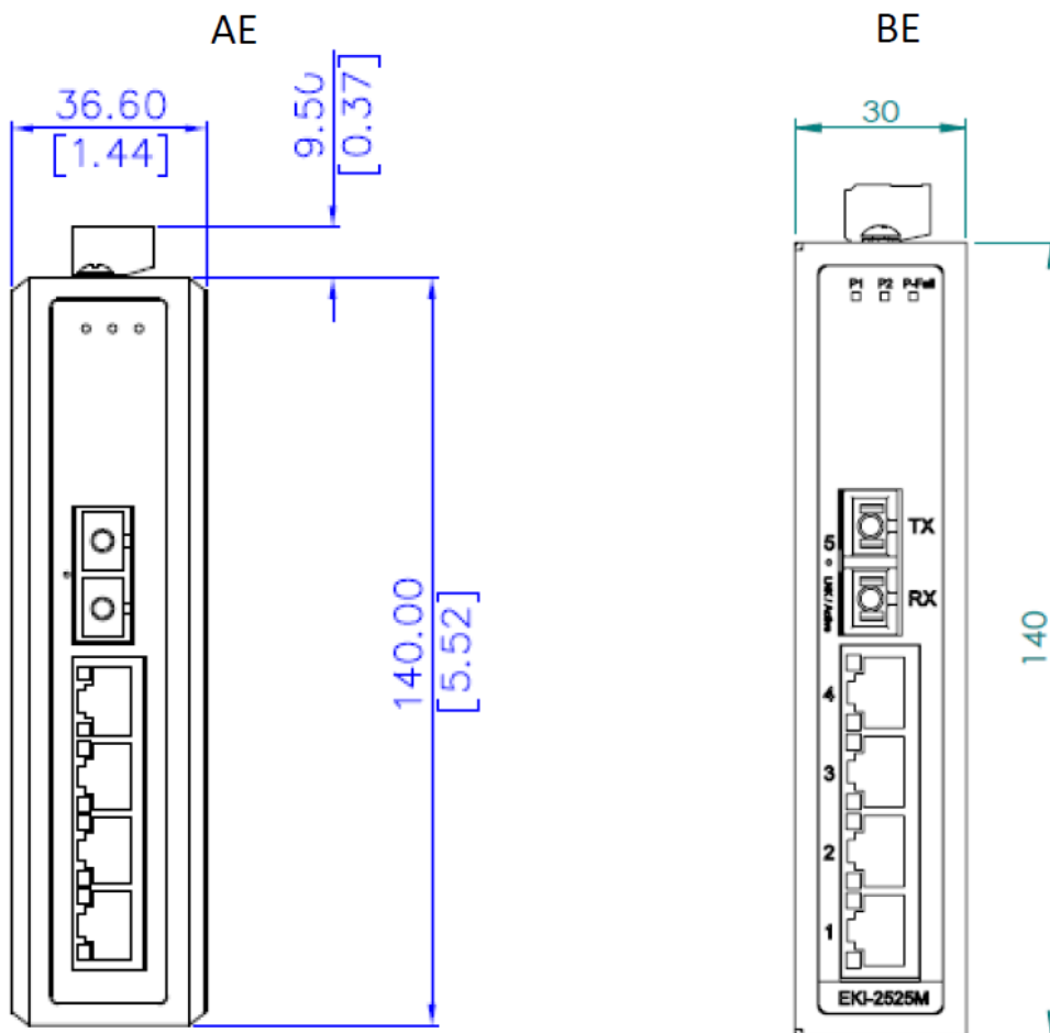
EKI-2525M/S-AE、及びEKI-2525M/S-BE寸法差分図
