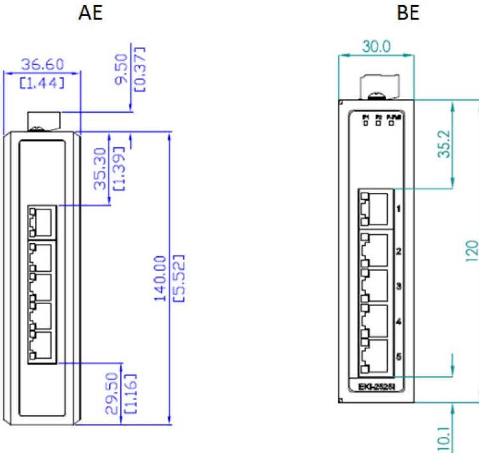
EKI-2525-AE、及びEKI-2525-BE寸法差分図
